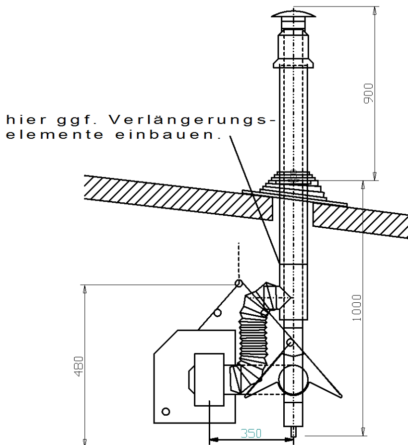
Abgas-/Frischluftführung IT-DR LAS DN 100/150
